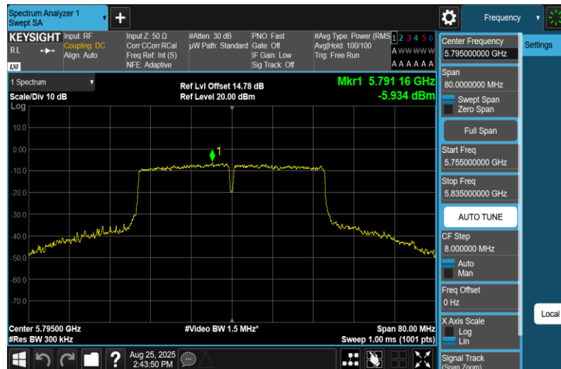
11N40MIMO-Ant1-5795-PASS
