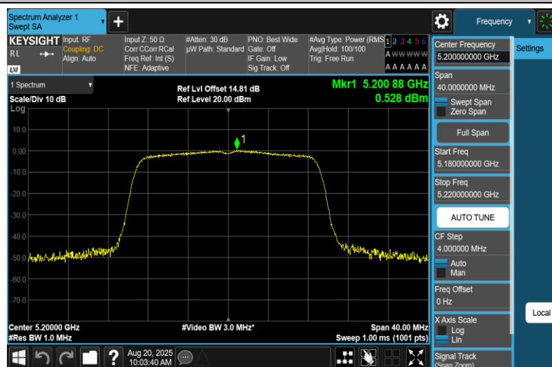
11N20MIMO-Ant1-5200-PASS
