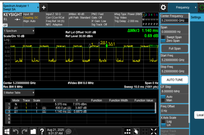
NTNV-11AC40MIMO-Ant1-5230
