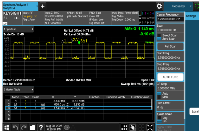
NTNV-11N40MIMO-Ant1-5795
