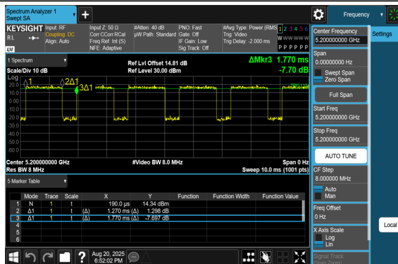
NTNV-11AC20MIMO-Ant1-5200
