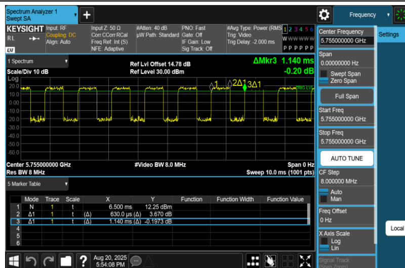
NTNV-11N40MIMO-Ant1-5755
