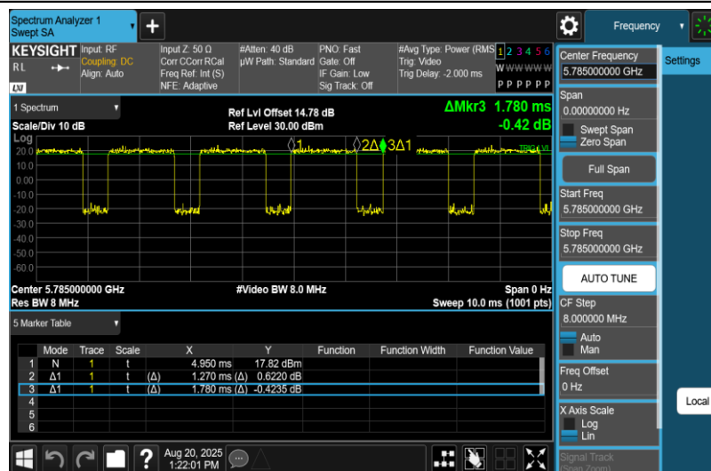
NTNV-11N20MIMO-Ant1-5785
