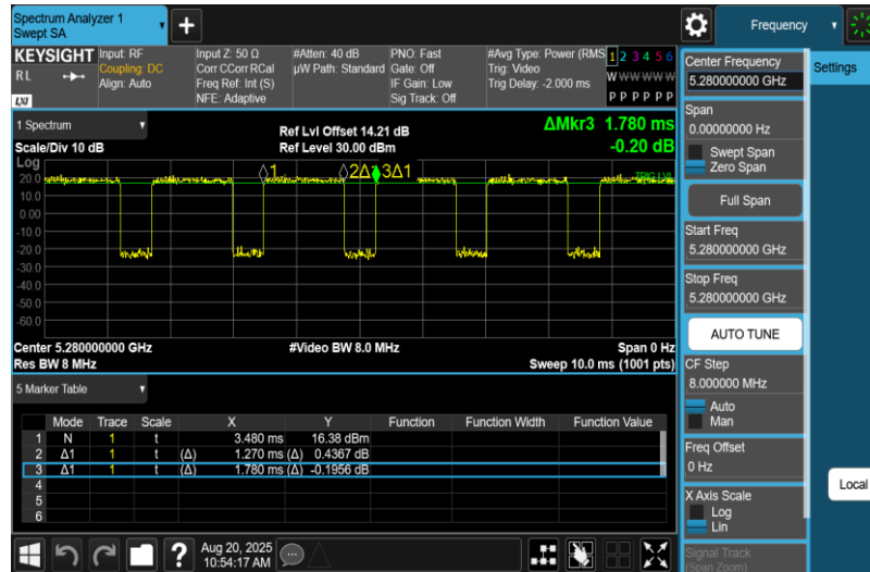
NTNV-11N20MIMO-Ant2-5280
