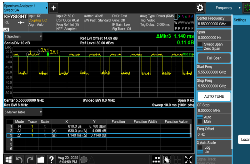
NTNV-11N40MIMO-Ant1-5550
