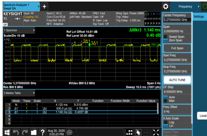
NTNV-11N40MIMO-Ant1-5270
