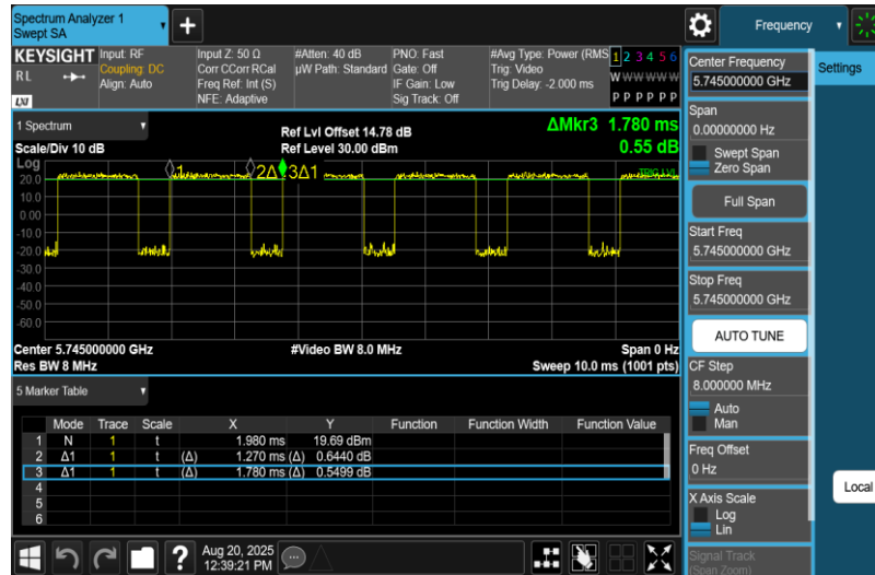
NTNV-11N20MIMO-Ant1-5745
