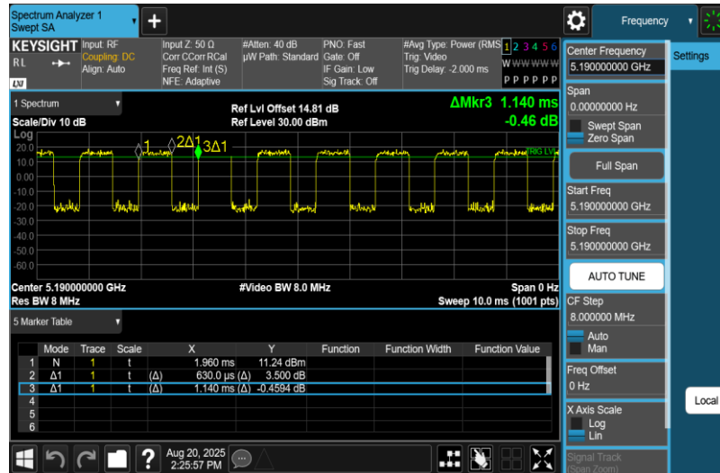
NTNV-11N40MIMO-Ant1-5190
