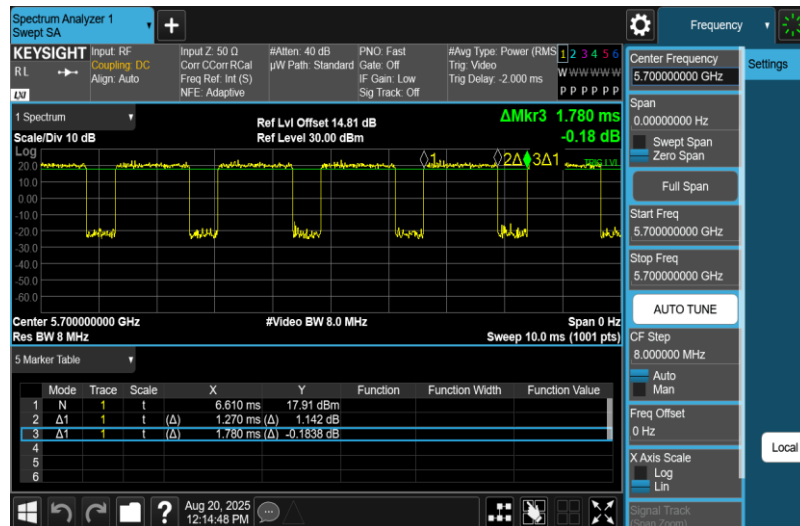
NTNV-11N20MIMO-Ant1-5700
