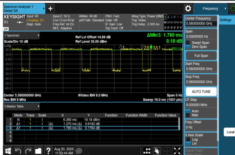
NTNV-11N20MIMO-Ant1-5580
