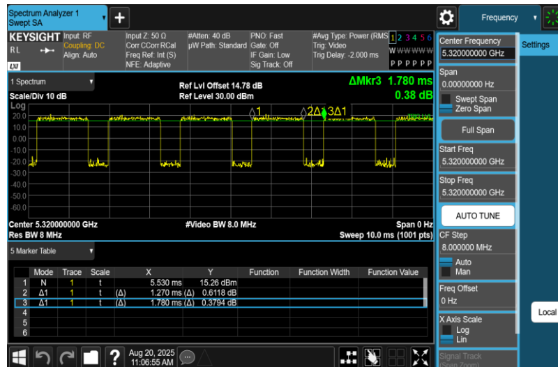
NTNV-11N20MIMO-Ant1-5320
