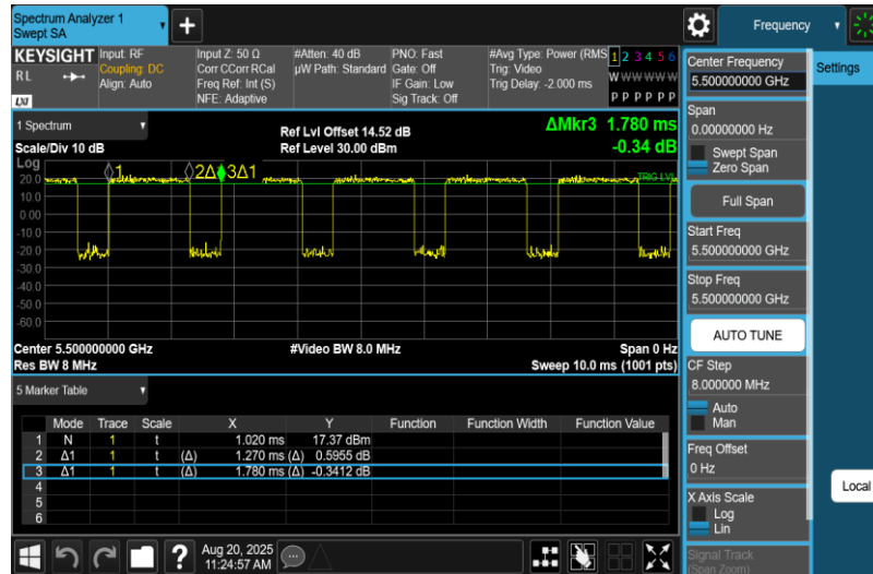
NTNV-11N20MIMO-Ant1-5500
