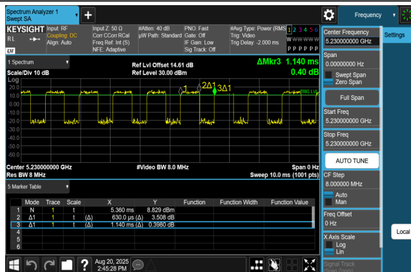
NTNV-11N40MIMO-Ant1-5230
