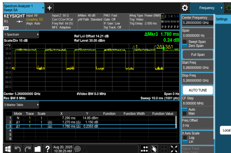
NTNV-11N20MIMO-Ant2-5260
