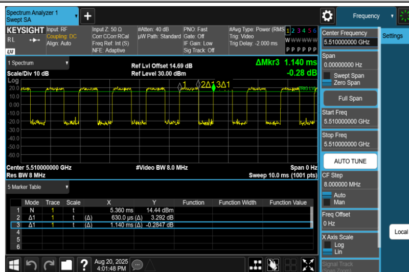
NTNV-11N40MIMO-Ant1-5510
