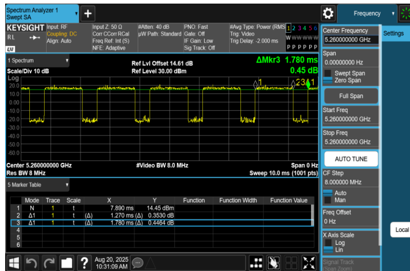
NTNV-11N20MIMO-Ant1-5260
