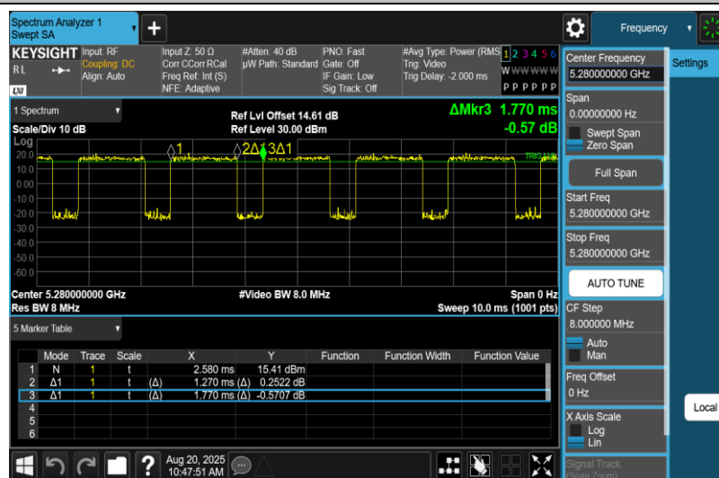
NTNV-11N20MIMO-Ant1-5280
