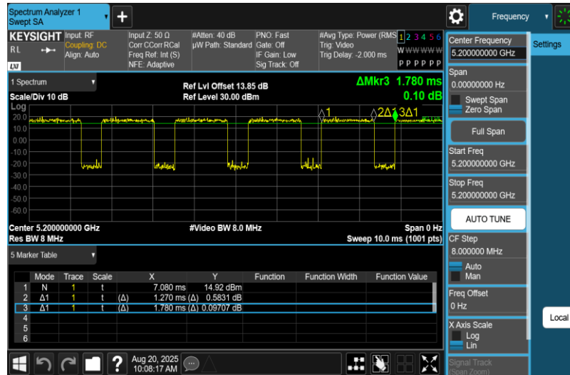
NTNV-11N20MIMO-Ant2-5200
