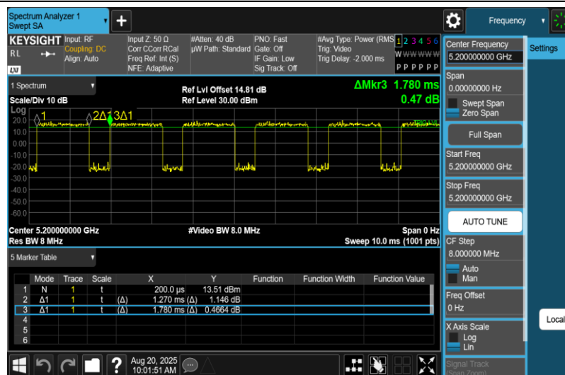
NTNV-11N20MIMO-Ant1-5200
