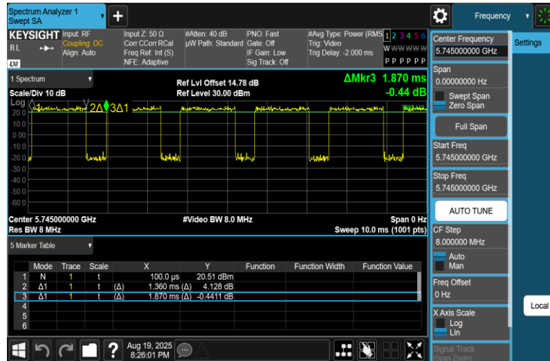
NTNV-11A-Ant1-5745
