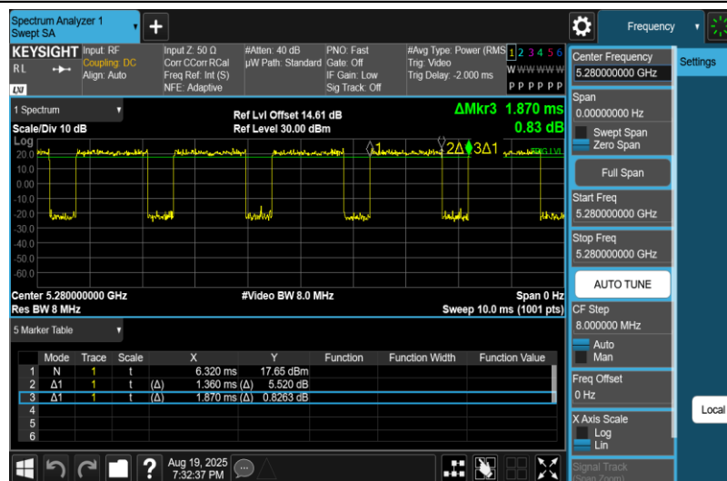
NTNV-11A-Ant1-5280
