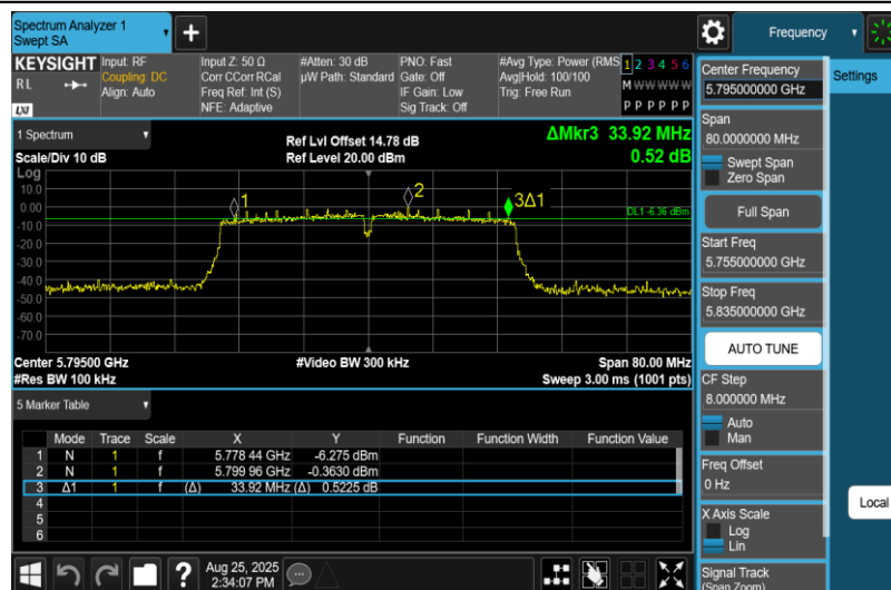
11N40MIMO-Ant1-5795-PASS
