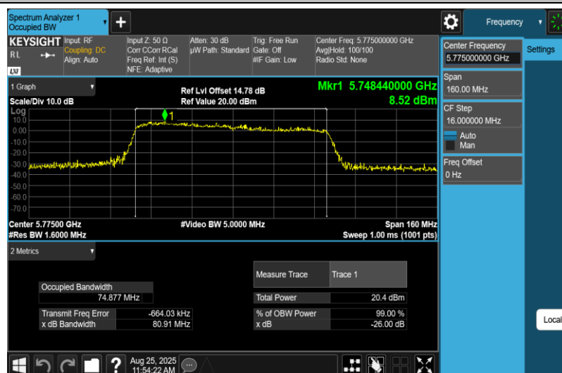
11AC80MIMO-Ant1-5775
