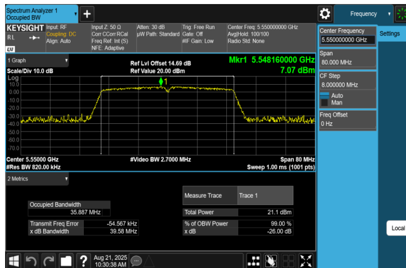
11AC40MIMO-Ant1-5550
