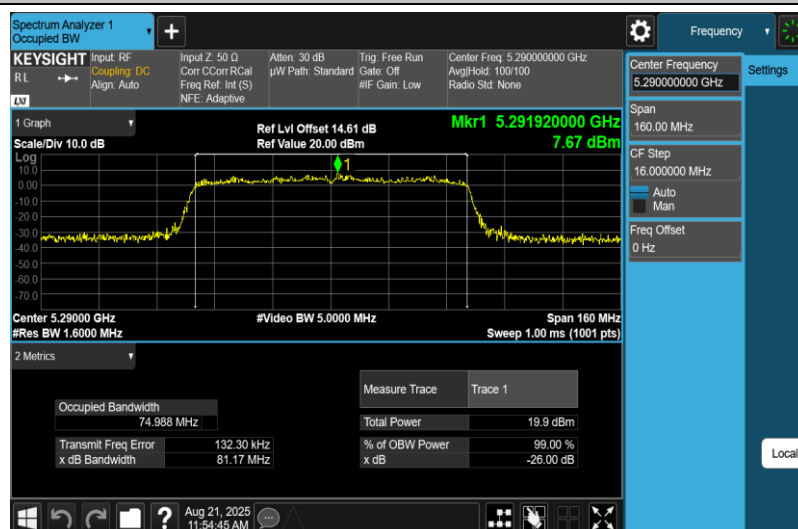
11AC80MIMO-Ant1-5290
