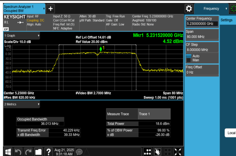
11AC40MIMO-Ant1-5230
