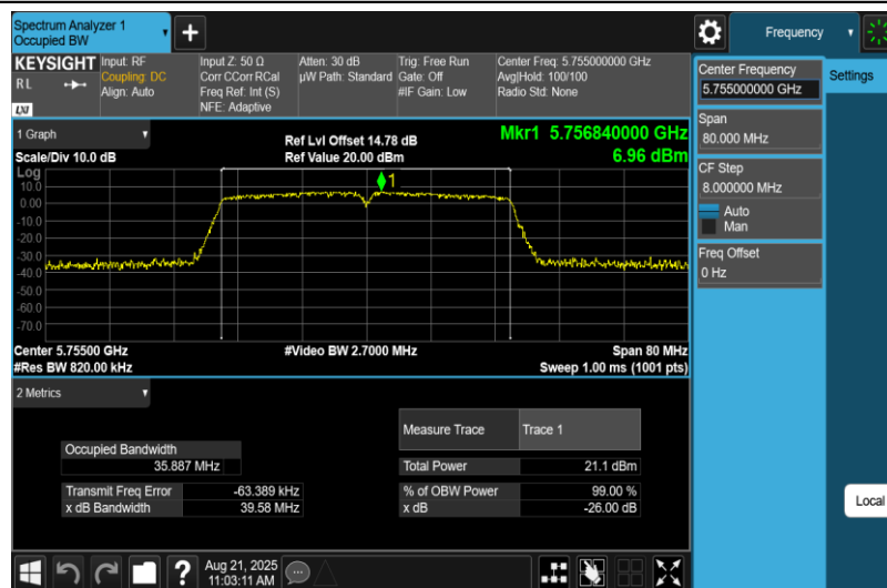
11AC40MIMO-Ant1-5755
