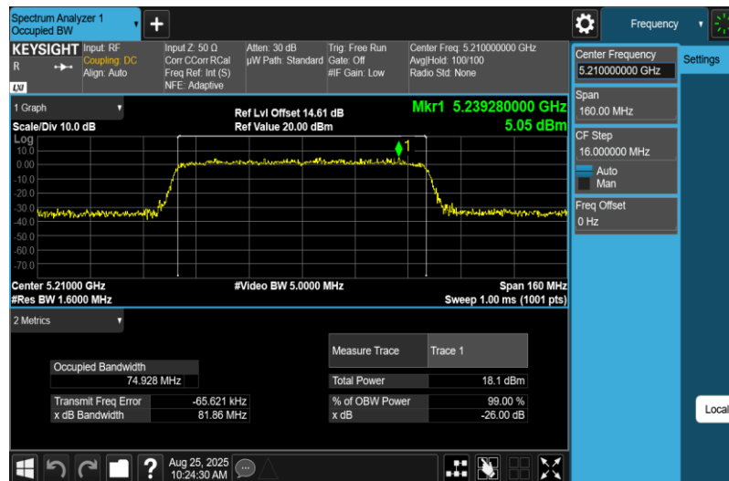
11AC80MIMO-Ant1-5210
