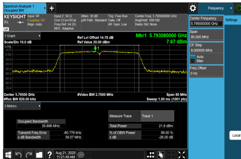
11AC40MIMO-Ant1-5795
