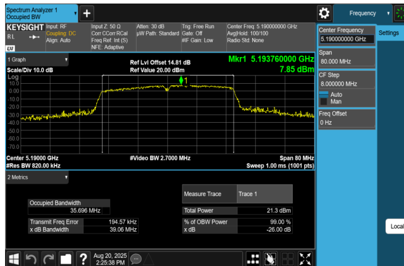
11N40MIMO-Ant1-5190
