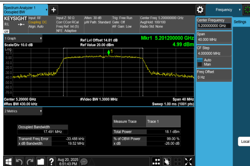
11AC20MIMO-Ant1-5200
