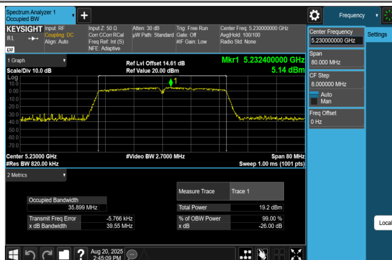
11N40MIMO-Ant1-5230
