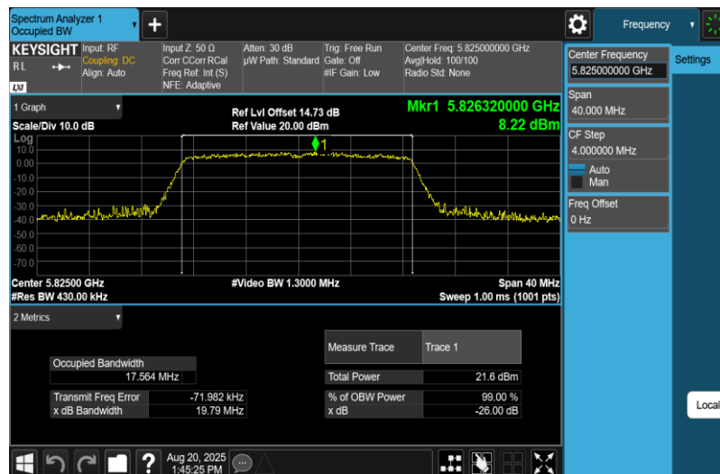
11N20MIMO-Ant1-5825
