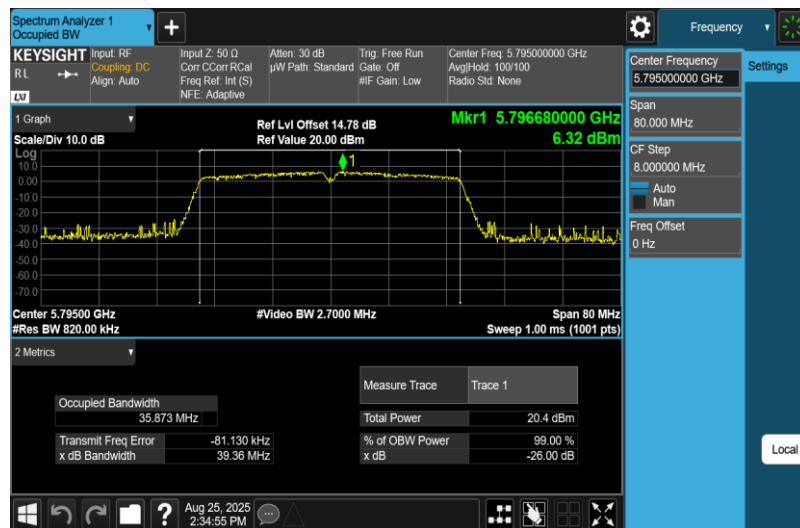
11N40MIMO-Ant1-5795
