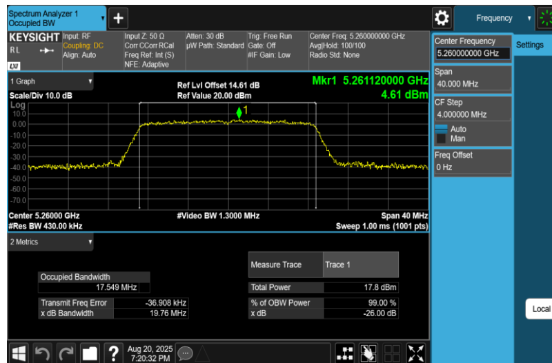
11AC20MIMO-Ant1-5260
