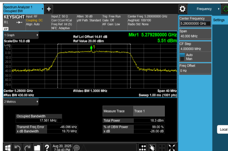
11AC20MIMO-Ant1-5280
