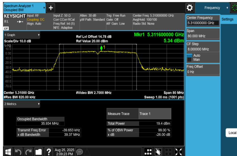
11N40MIMO-Ant1-5310
