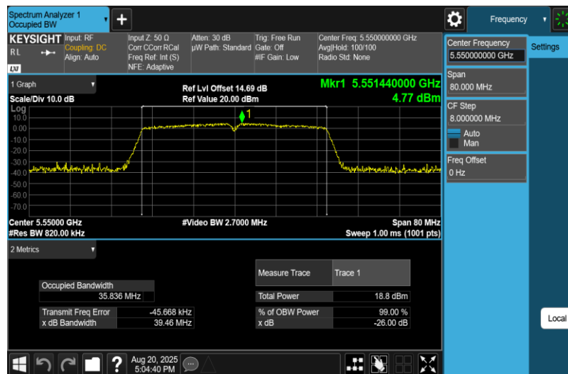
11N40MIMO-Ant1-5550
