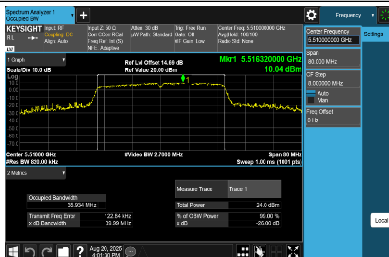
11N40MIMO-Ant1-5510
