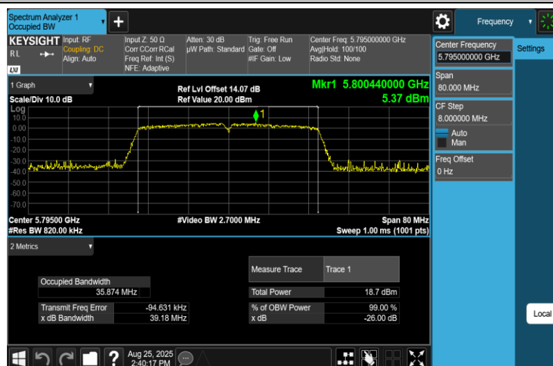
11N40MIMO-Ant2-5795
