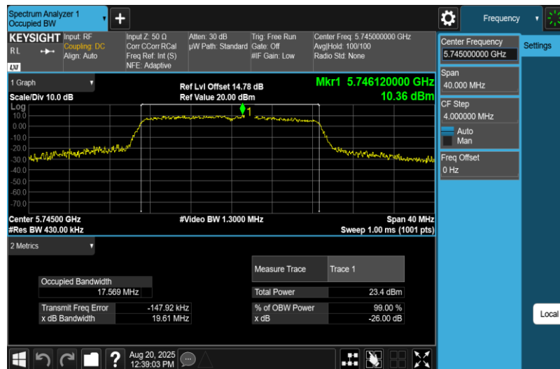
11N20MIMO-Ant1-5745
