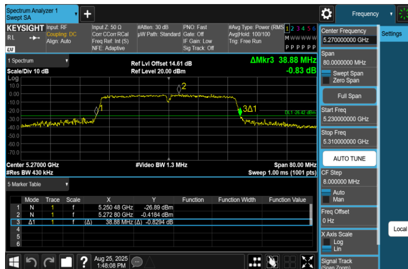
11AC40MIMO-Ant1-5270
