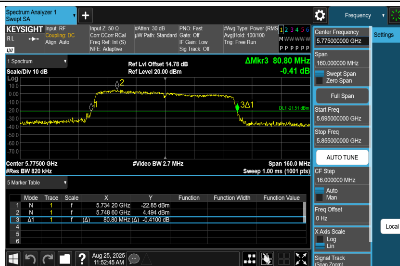
11AC80MIMO-Ant1-5775
