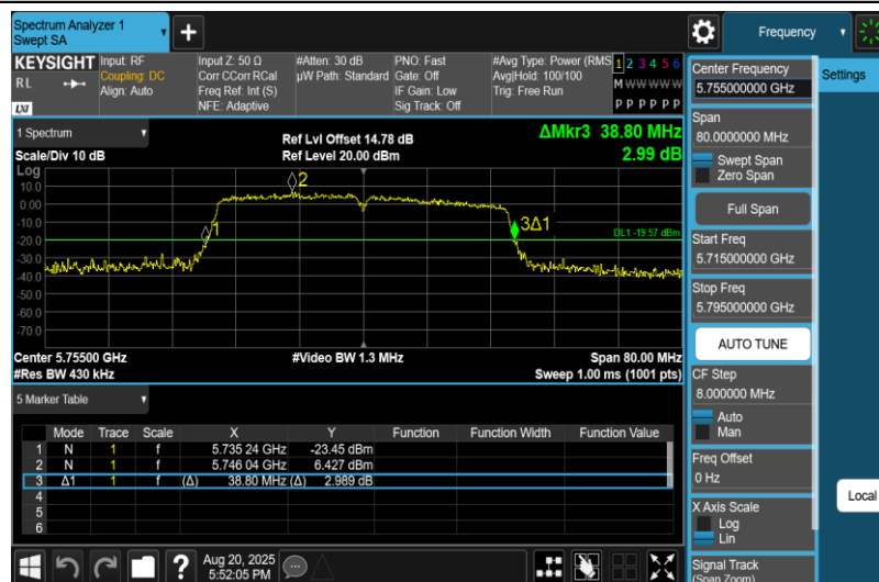
11N40MIMO-Ant1-5755
