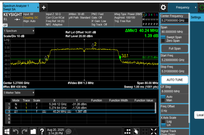
11N40MIMO-Ant1-5270
