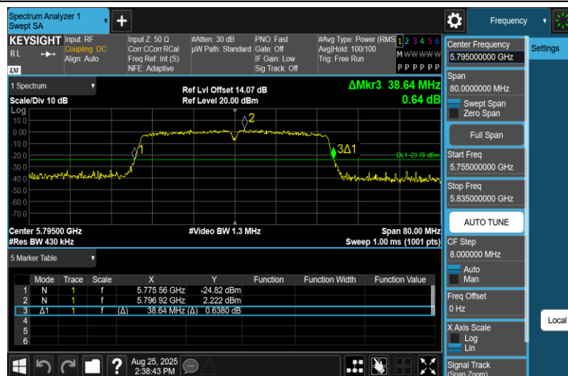
11N40MIMO-Ant2-5795
