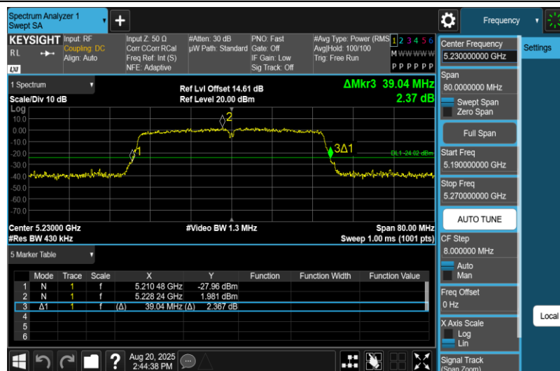
11N40MIMO-Ant1-5230
