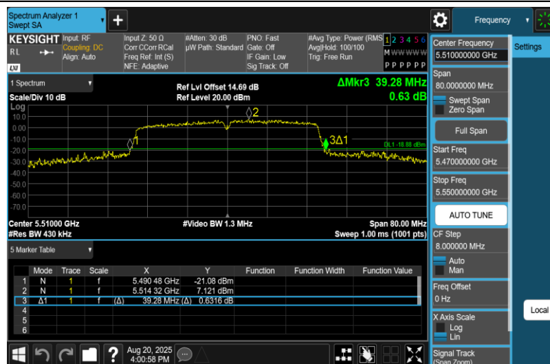
11N40MIMO-Ant1-5510
