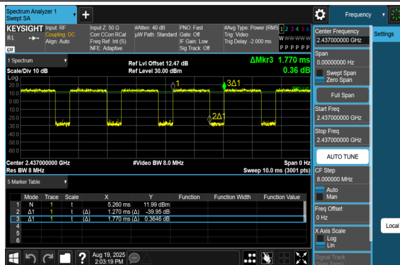
NTNV-11N20MIMO-Ant1-2437
