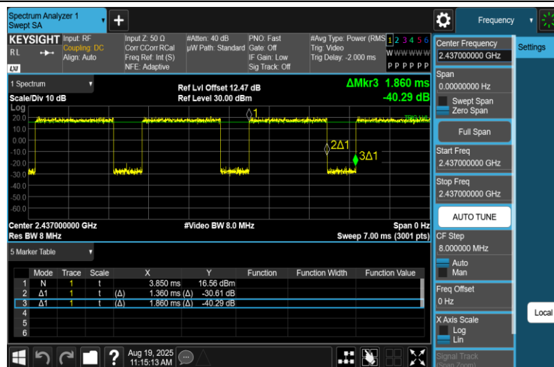
NTNV-11G-Ant1-2437
