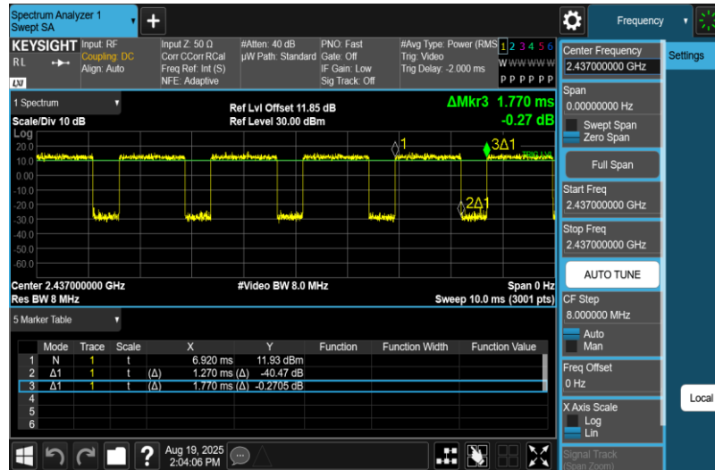
NTNV-11N20MIMO-Ant2-2437
