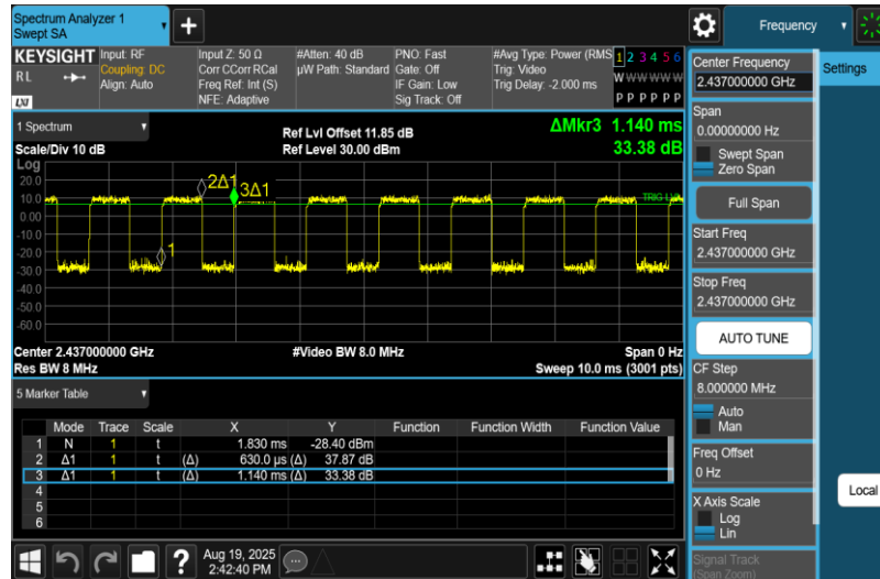
NTNV-11N40MIMO-Ant2-2437
