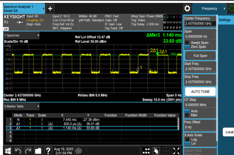
NTNV-11N40MIMO-Ant1-2437
