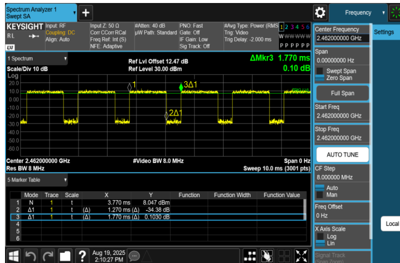
NTNV-11N20MIMO-Ant1-2462
