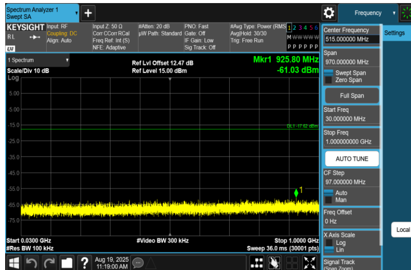
11G-Ant1-2437-30~1000-PASS
