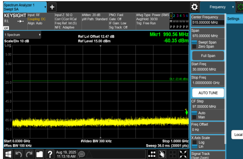
11G-Ant1-2412-30~1000-PASS
