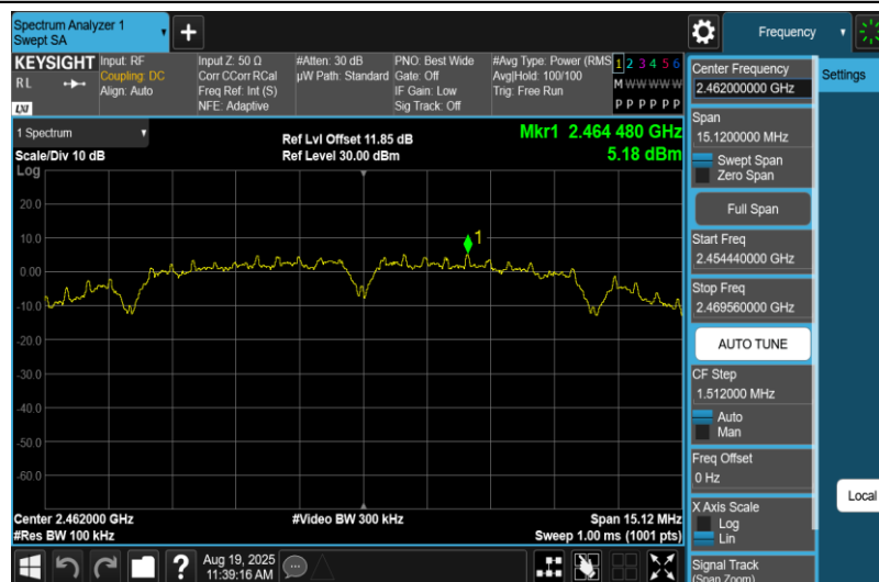
11B-Ant2-2462-PASS
