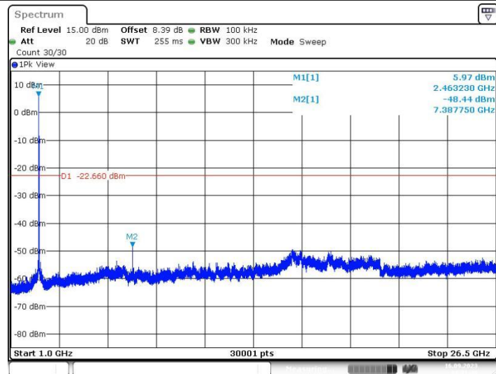
11B_Ant2_2462_1000~26500
