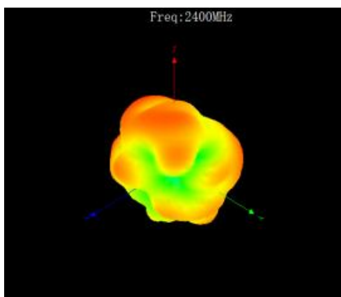
2400MHZ
