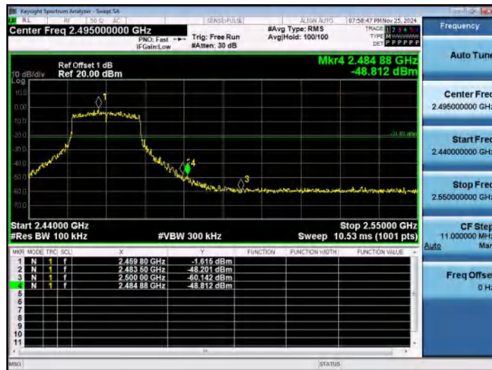
11AX20ISO-Ant1-2462-PASS
