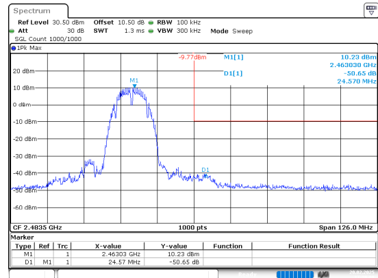
802.11b_2462MHz
