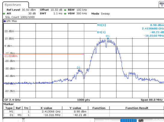
802.11b_2412MHz
