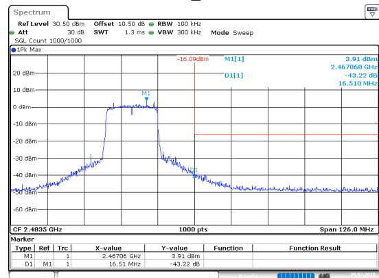
802.11n20_2462MHz
