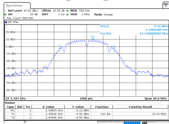
802.11b_2437MHz_Chain 0
