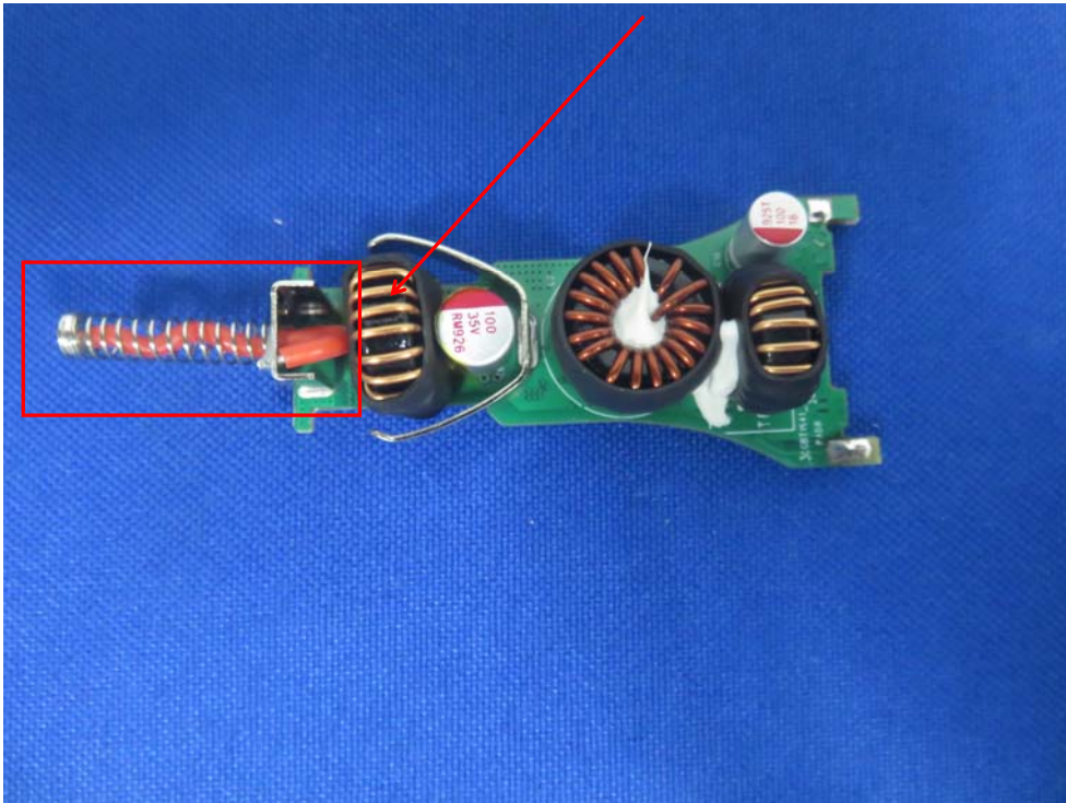
FM ANT
