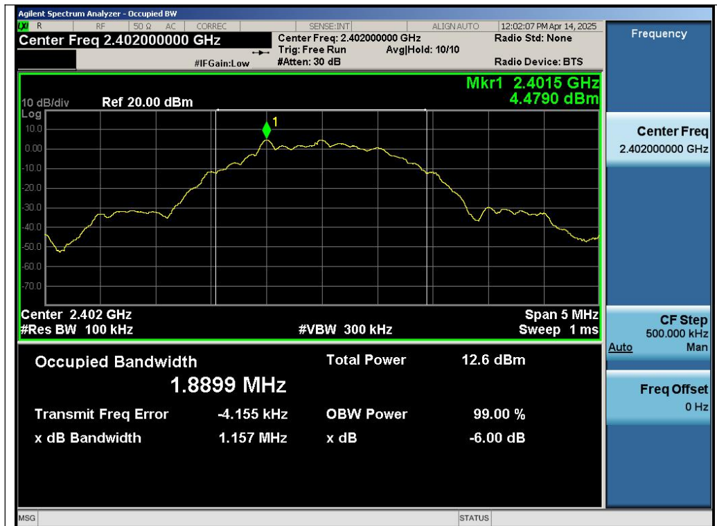
Test_Graph_GFSK_ANT1_2402_2Mbps_DTSBW
