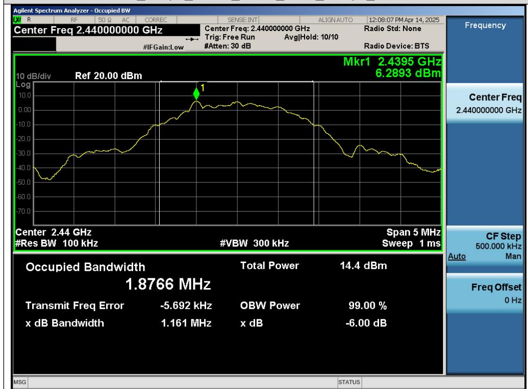
Test_Graph_GFSK_ANT1_2440_2Mbps_DTSBW
