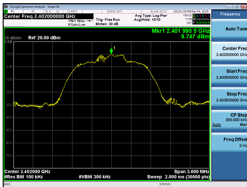
Test_Graph_EDR_ANT1_2402_2Mbps_Reference Level
