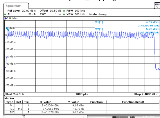
\pi/4 -DQPSK_Hopping
