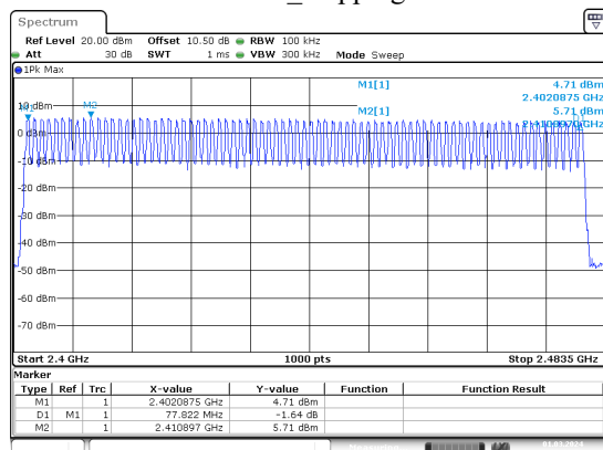
GFSK_Hopping
