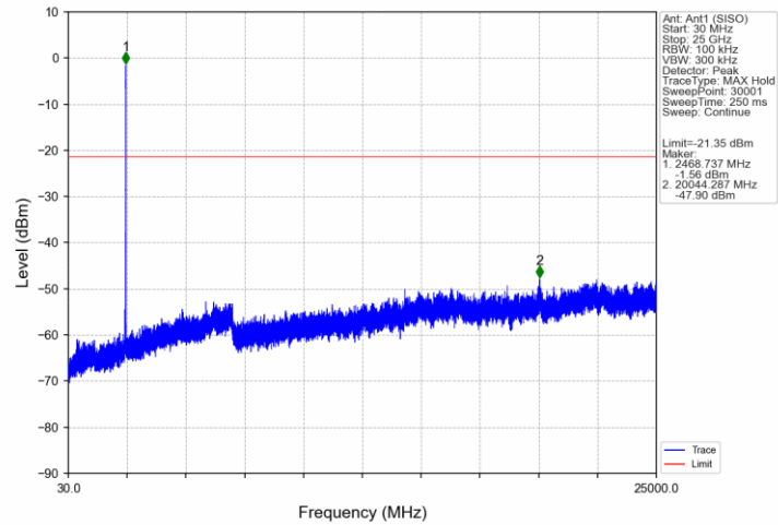
802.11ax(HEW20)_HCH_2462MHz_RU106_54_Ant1 (SISO)_NTNV
