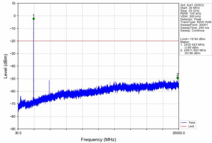
802.11ax(HEW40)_MCH_2437MHz_RU106_54_Ant1 (SISO)_NTNV
