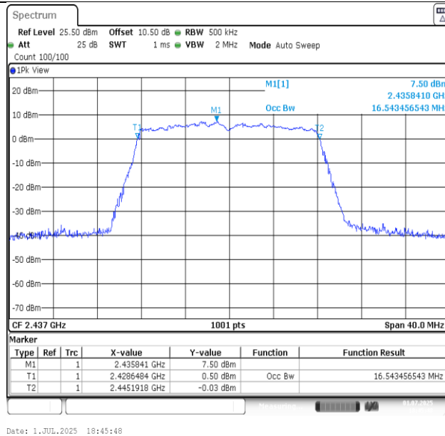
11G-Ant1-2437
