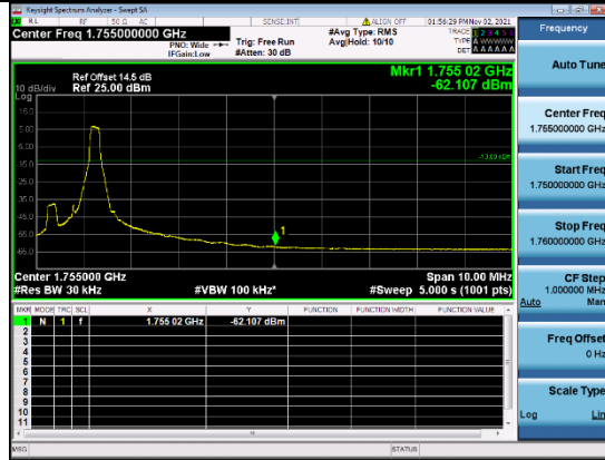
B4-5M-High CH-CSE-1-Q16-1 RB 0
