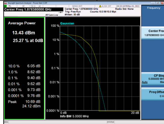
B2-5M-Mid CH-PAPR-QPSK
