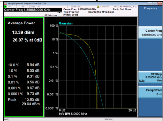
B2-5M-Low CH-PAPR-QPSK
