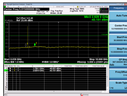
B2-20M-High CH-CSE-2-Q16-1 RB 0
