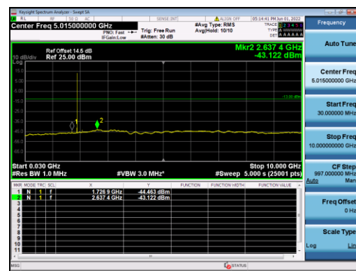
B2-5M-High CH-CSE-2-Q16-1 RB 0
