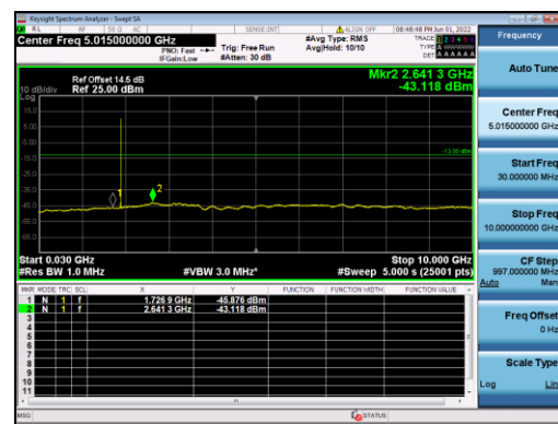
B2-3M-High CH-CSE-2-Q16-1 RB 0
