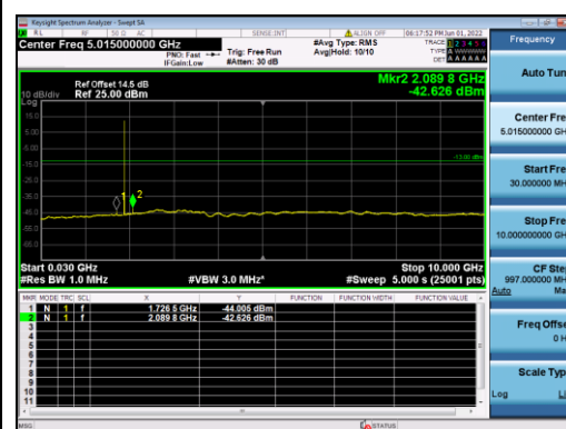
B2-15M-High CH-CSE-2-Q16-1 RB 0
