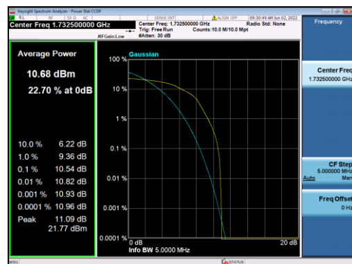
B4-1.4M-Mid CH-PAPR-Q16
