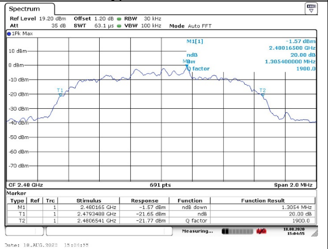
Modulation type: \pi/4 DQPSK 2480MHz
