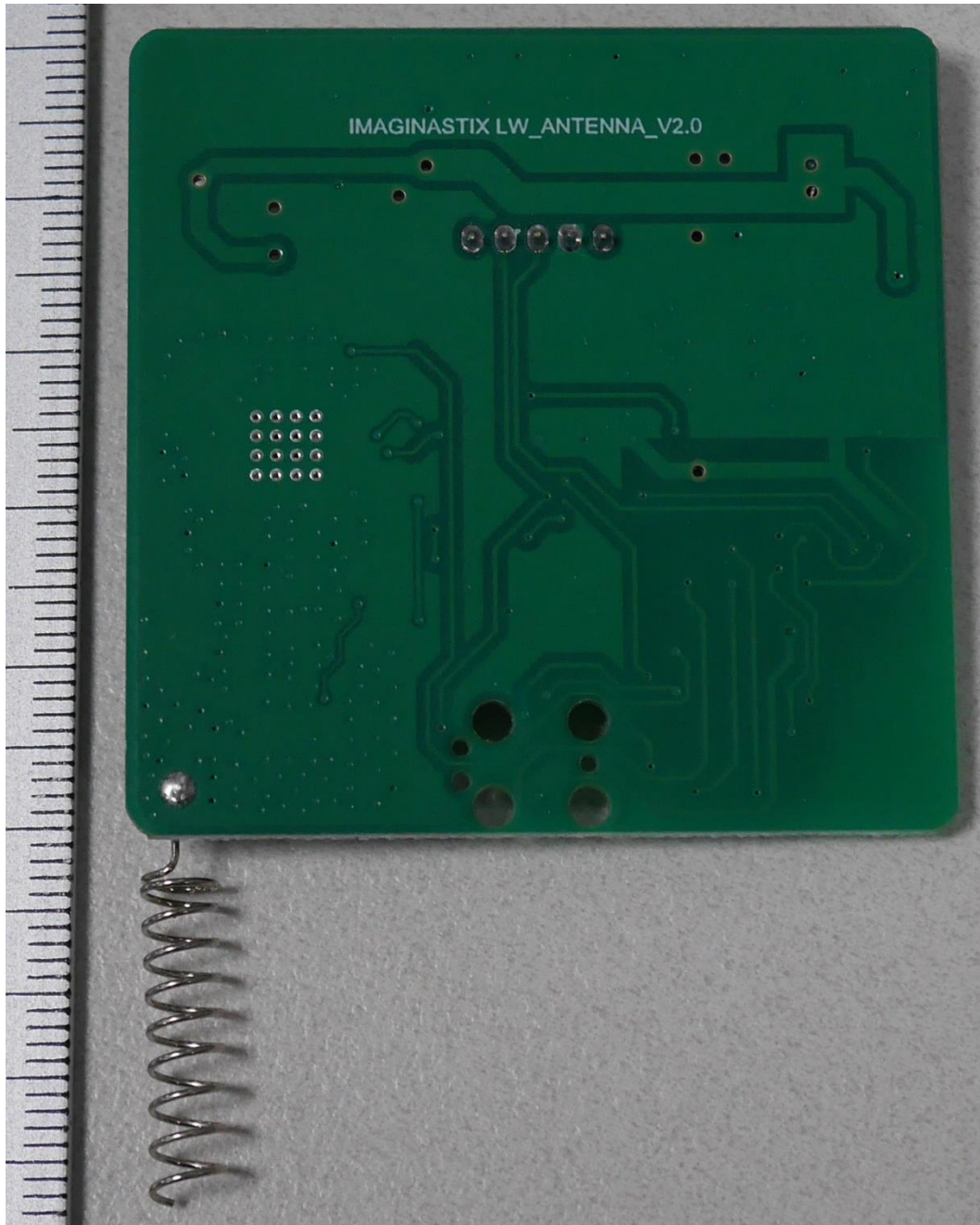
PCB bottom
