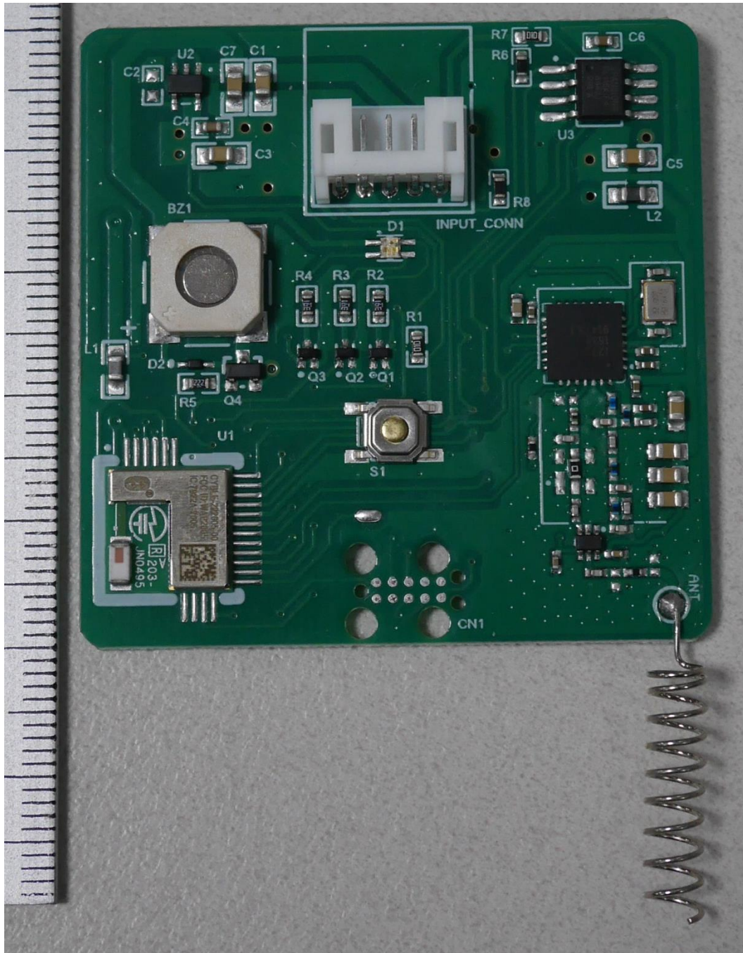
PCB Top
