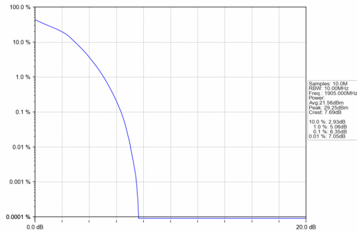
Band2 10MHz 16QAM HCH 1905MHz RB 50 0 NTNV
