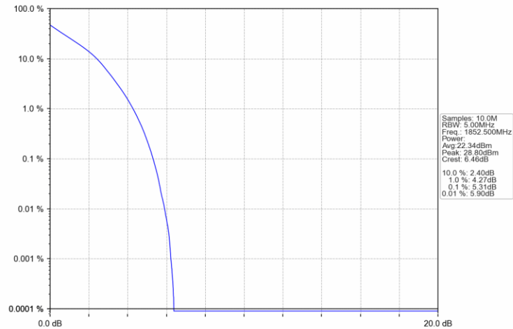
Band2 5MHz QPSK LCH 1852.5MHz RB 25 0 NTN
