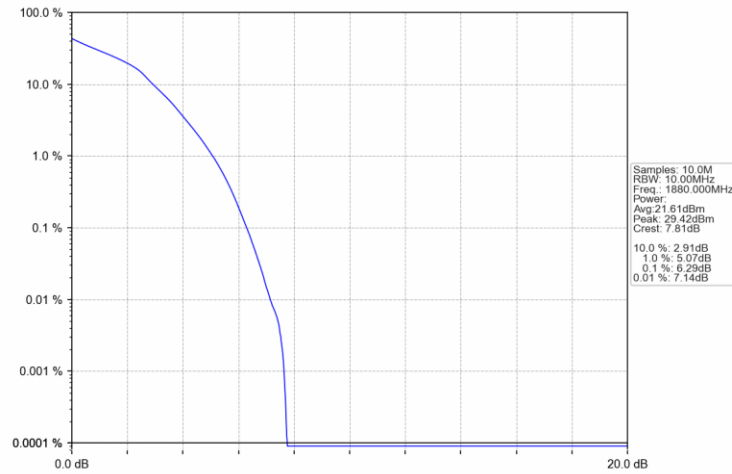
Band2 10MHz 16QAM MCH 1880MHz RB 50 0 NTNV
