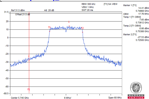
802.11ac(VHT20)_Chain3 / CH149
