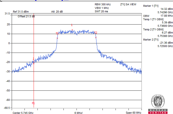
802.11ac(VHT20)_Chain3 / CH149
