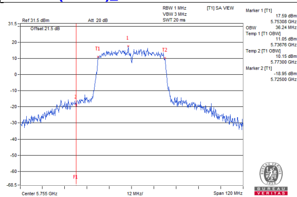
802.11ac(VHT40)_Chain3 / CH151
