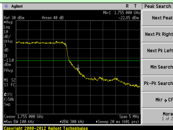
10MHz Bandwidth (RB size:12# RB offset:13#)
