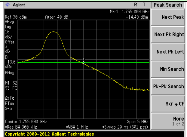
20MHz Bandwidth (RB size:1# RB offset:24#)
