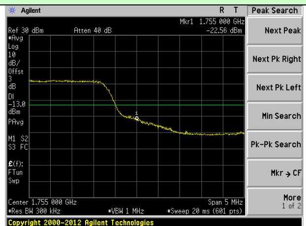
20MHz Bandwidth (RB size:25# RB offset:0#)
