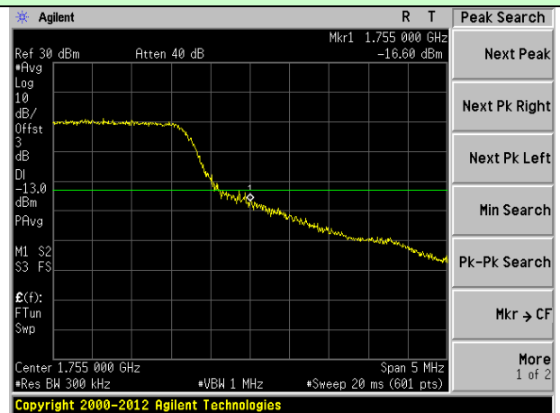
20MHz Bandwidth (RB size:12# RB offset:13#)
