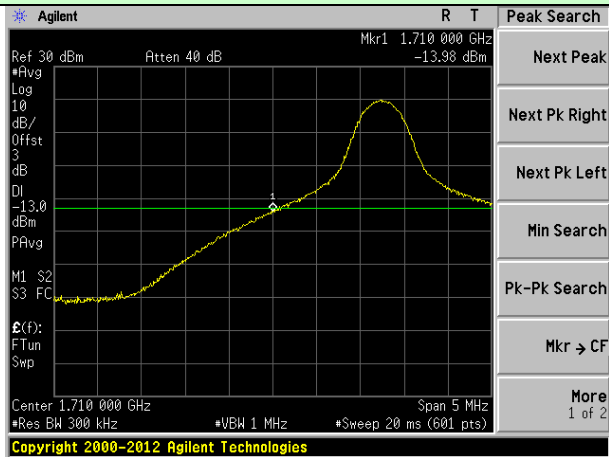
20MHz Bandwidth (RB size:1# RB offset:0#)
