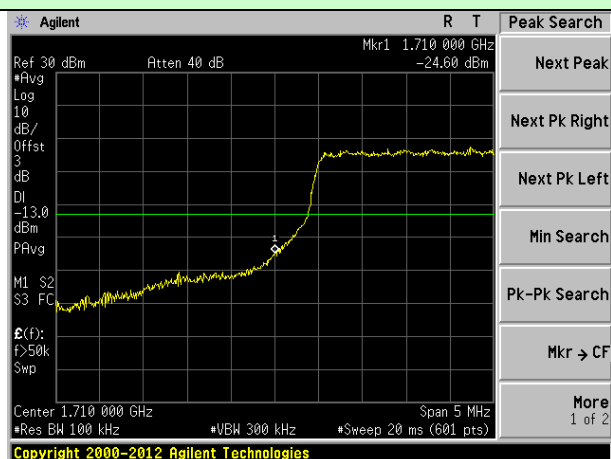
10MHz Bandwidth (RB size:12# RB offset:0#)
