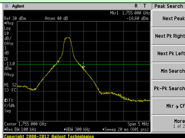
10MHz Bandwidth (RB size:1# RB offset:24#)
