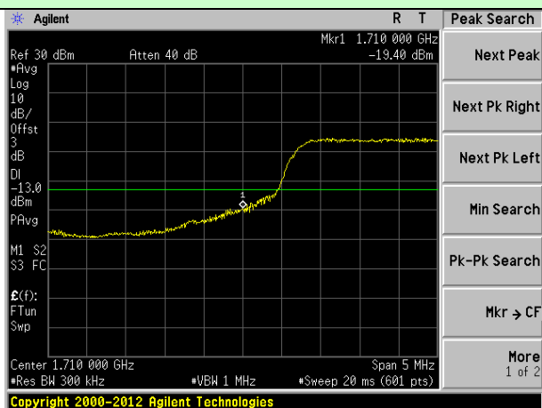
20MHz Bandwidth (RB size:25# RB offset:0#)
