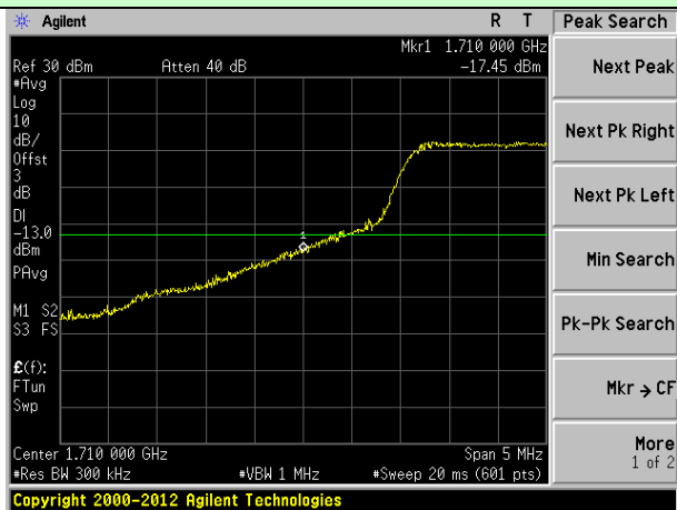
20MHz Bandwidth (RB size:12# RB offset:0#)
