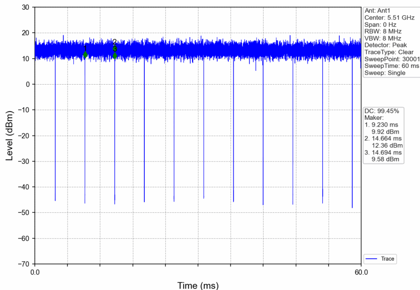
802.11ax(HEW40)_LCH_5510MHz_RU484_Left_Ant1_NTNV
