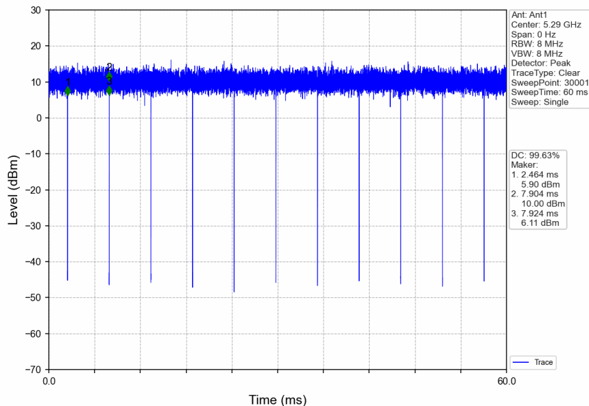
802.11ax(HEW80)_MCH_5290MHz_RU996_Left_Ant1_NTNV
