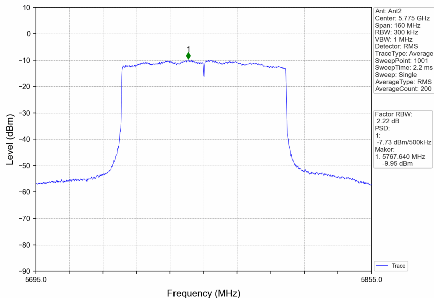
802.11ax(HEW80)_MCH_5775MHz_RU996_Left_Ant2_NTNV
