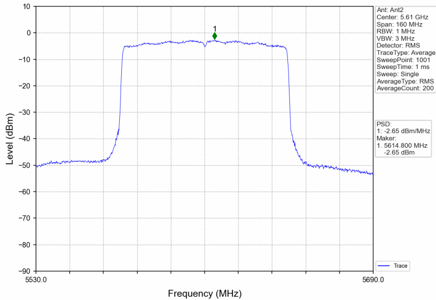
802.11ax(HEW80)_HCH_5610MHz_RU996_Left_MIMO_NTNV
