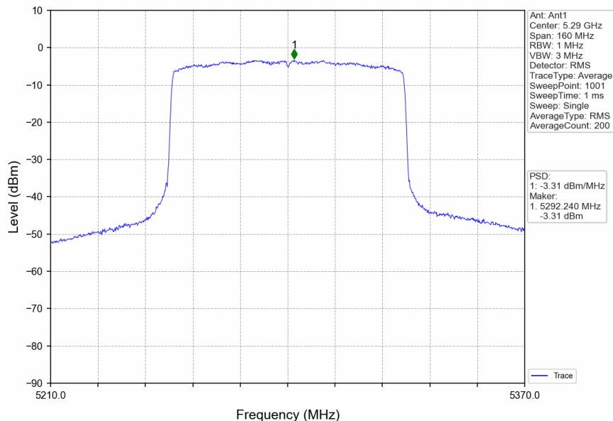
802.11ax(HEW80)_MCH_5290MHz_RU996_Left_Ant1_NTNV
