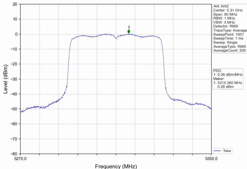
802.11ax(HEW40)_HCH_5310MHz_RU484_Left_Ant2_NTNV
