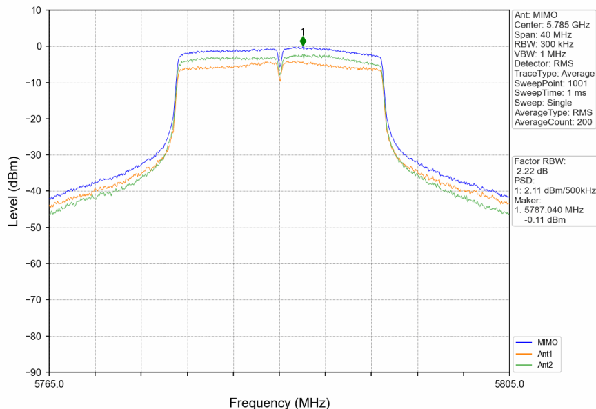
802.11n(HT20)_MCH_5785MHz_MIMO_NTNV
