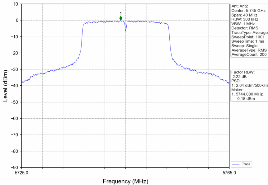
802.11a_LCH_5745MHz_Ant2_NTNV
