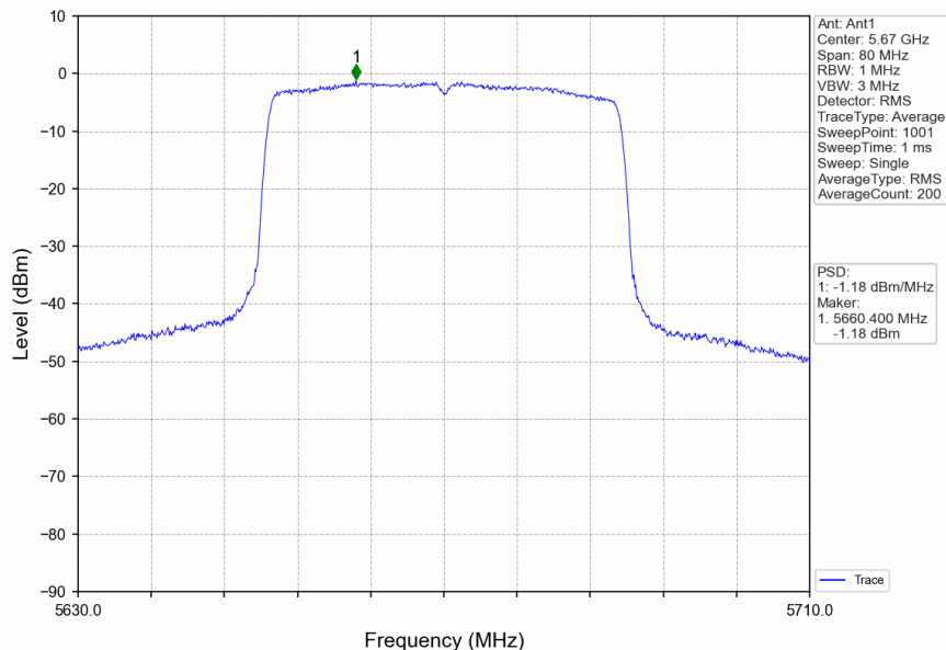
802.11ax(HEW40)_HCH_5670MHz_RU484_Left_Ant1_NTNV
