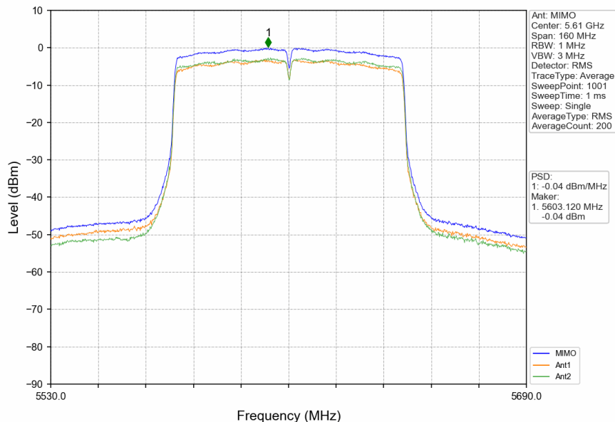
802.11ac(VHT80)_HCH_5610MHz_MIMO_NTNV
