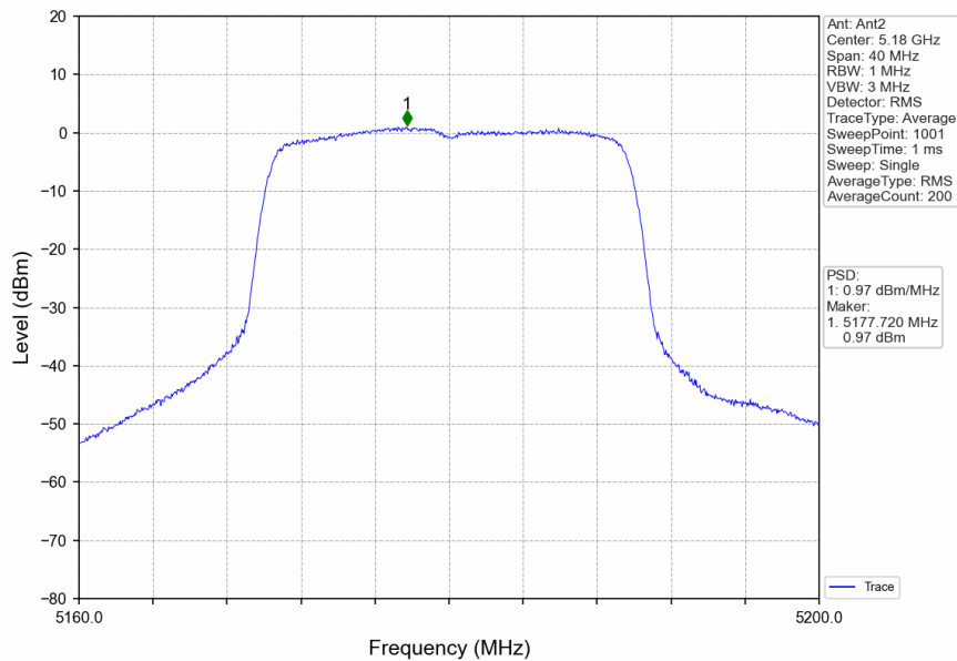
802.11ax(HEW20)_LCH_5180MHz_RU242_Left_Ant2_NTNV
