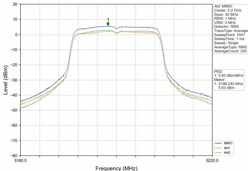
802.11n(HT20)_MCH_5200MHz_MIMO_NTNV
