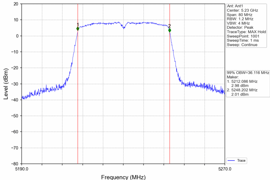
802.11n(HT40)_HCH_5230MHz_Ant1_NTNV
