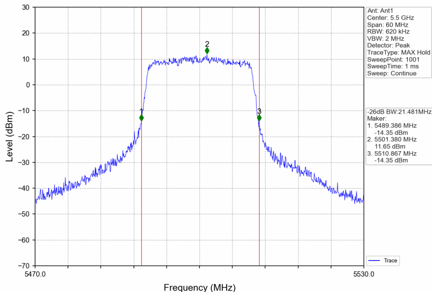
802.11ax(HEW20)_LCH_5500MHz_RU242_Left_Ant1_NTNV
