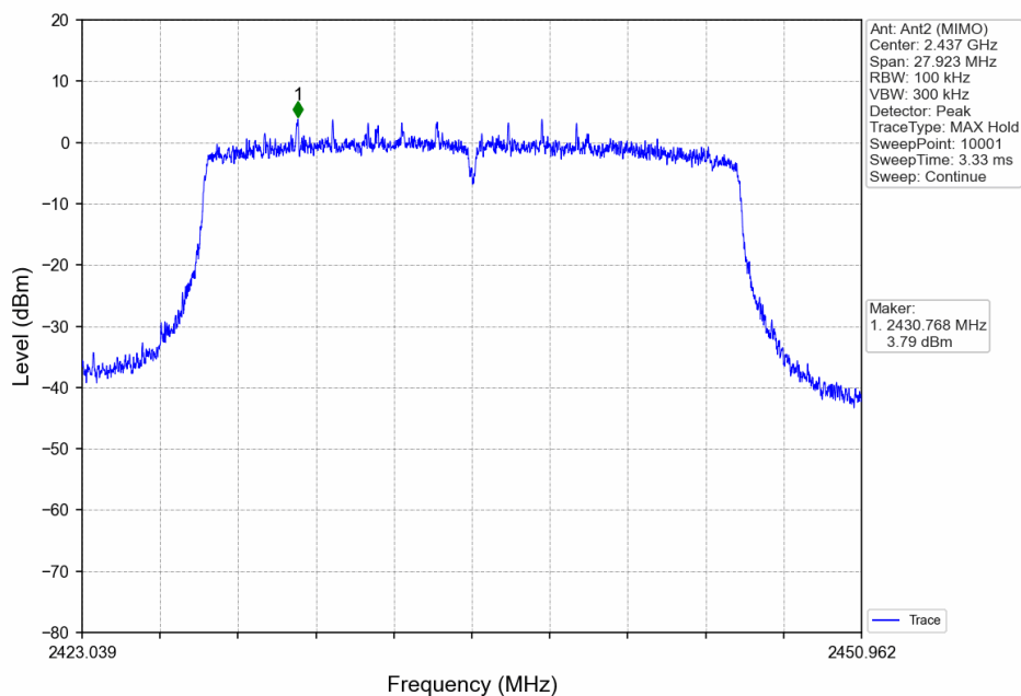
802.11ax(HEW20)_MCH_2437MHz_RU242_Left_Ant2 (MIMO)_NTNV
