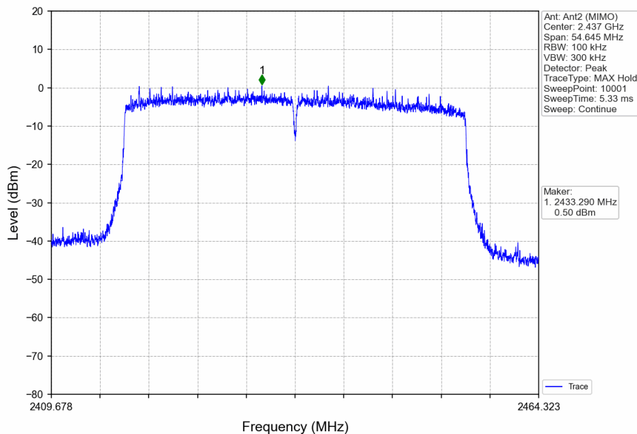
802.11ax(HEW40)_MCH_2437MHz_RU484_Left_Ant2 (MIMO)_NTNV
