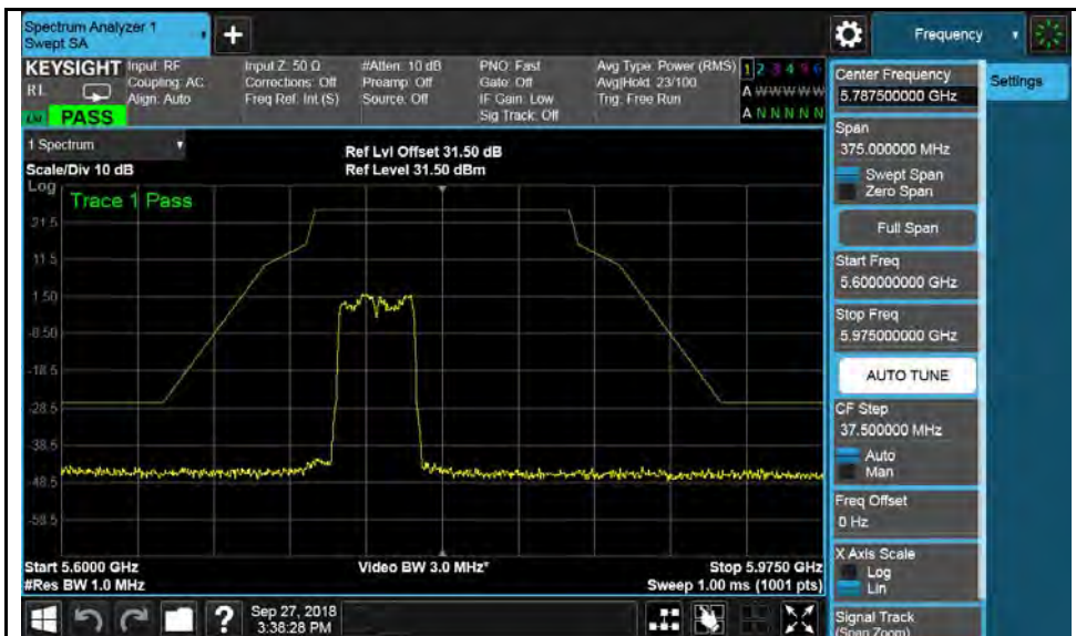
802.11ac-VHT40-5755MHz
