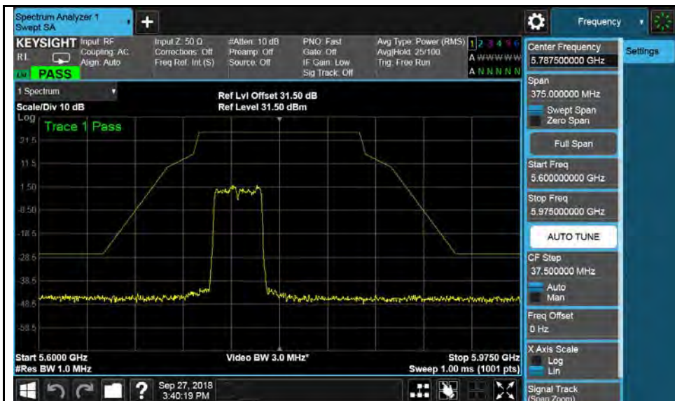
802.11ac-VHT40-5755MHz
