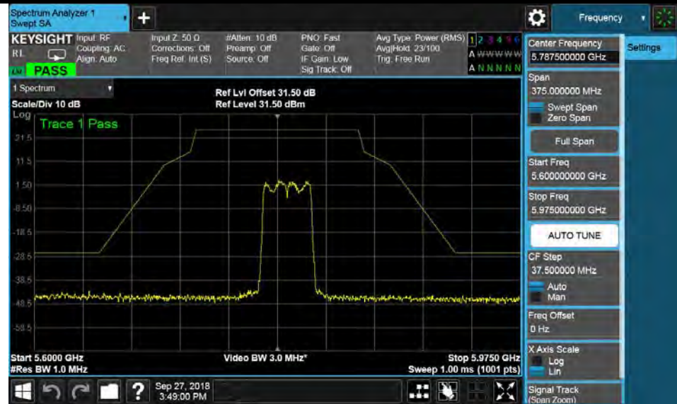
802.11ac-VHT40-5795MHz
