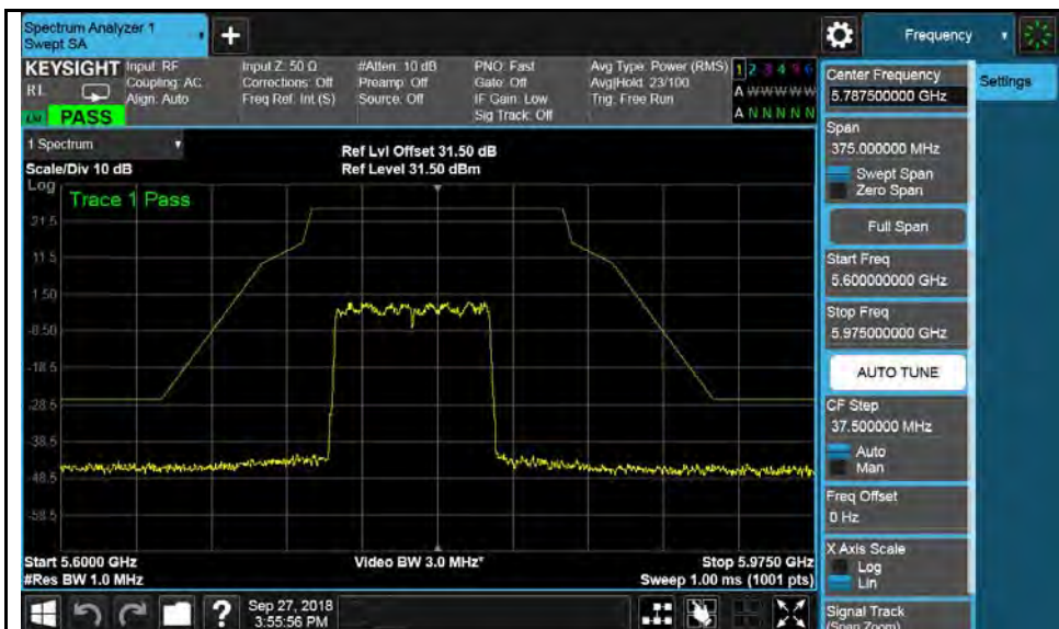
802.11ac-VHT80-5775MHz
