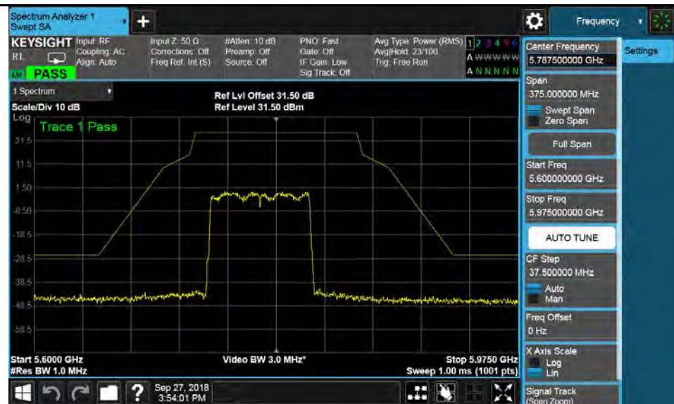
802.11ac-VHT80-5775MHz
