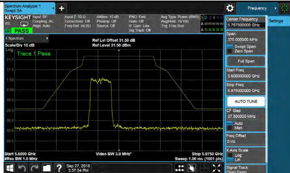
802.11ac-VHT40-5755MHz
