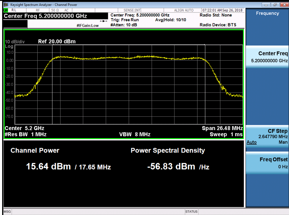
802.11ac20 5200M
