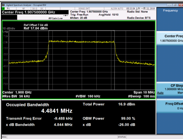
HCH_QPSK_25RB#0
