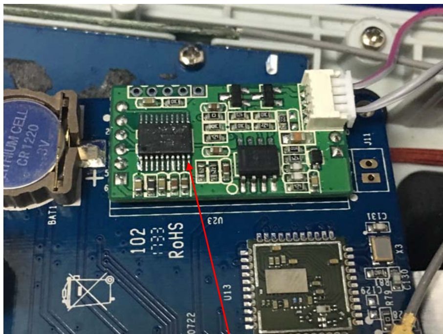
RFID MODULE
