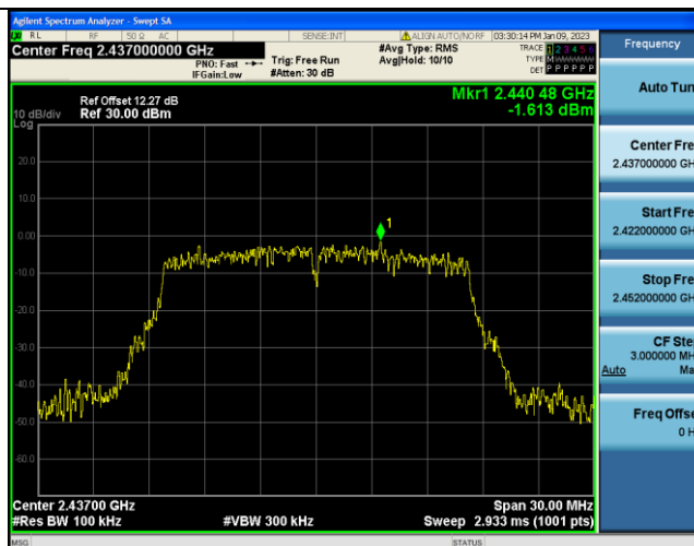
11G-Ant1-2437-30~1000~-1.61
