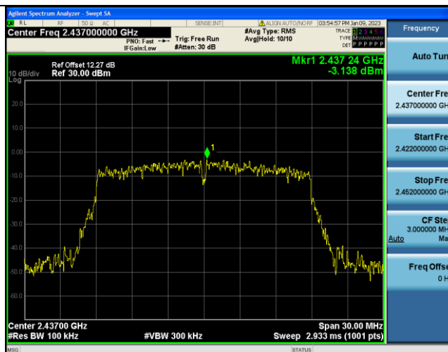
11N20SISO-Ant1-2437-30~1000--3.14
