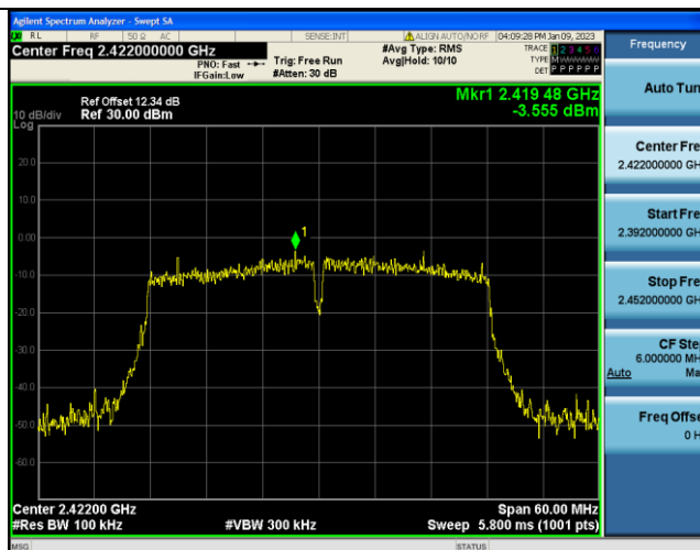
11N40SISO-Ant1-2422-30~1000--3.56
