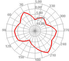
2450.000MHz E2
