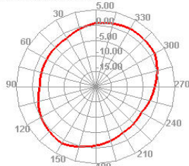
2450.000MHz H
