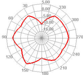
2450.000MHz E1
