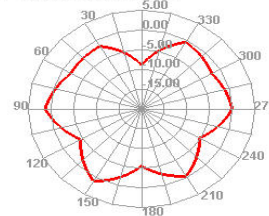
2400.000MHz E1
