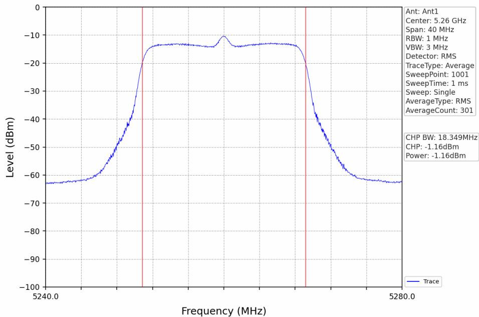
802.11n(HT20)_LCH_5260MHz_Ant1_NTNV
