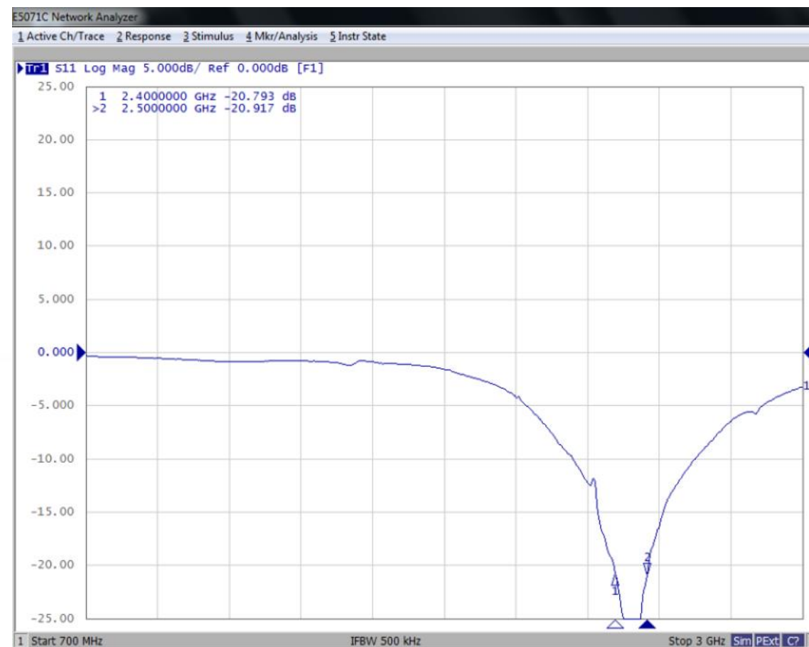
S-Parameter Test
