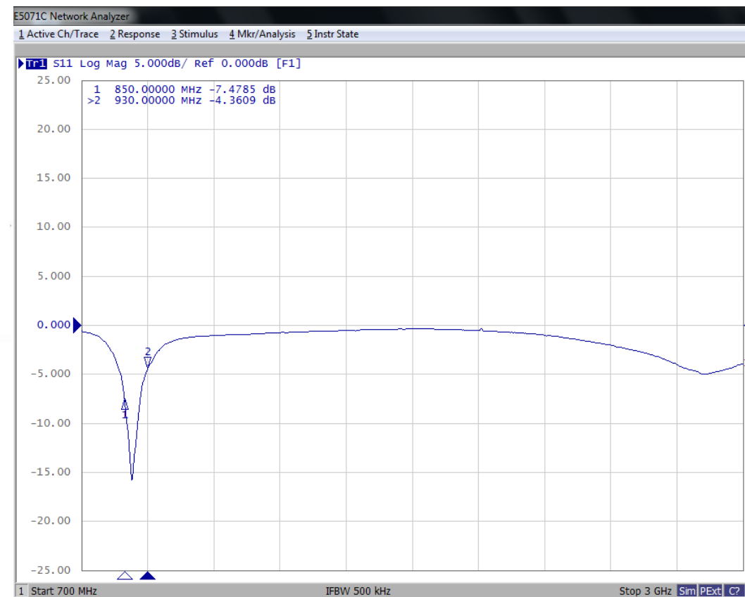
S-Parameter Test
